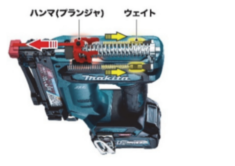
低反動機構 (カウンターウェイト方式)
